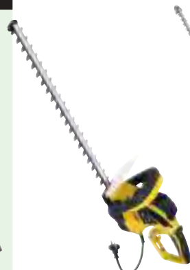
GARLAND CORTASETOS ELÉCTRICO 135314 Potencia 750W, peso 3,6 Kg, cuchilla de 73 cm de 24 mm entre dientes con engranajes en 2 escalones y asa rotable 90°.
