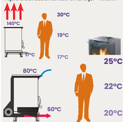
SUPRA STINA 23022581 7,3kW (5-15kW). 62,4 x 43,3 x 66,5 cm. Cuerpo de hierro fundido y patas de madera. Placas lat. de Vermiculita alta densidad. ø 150 mm. ø Aire 100 mm. Compatible hogares eficientes. Salida humos superior o posterior. Rendimiento 78%. Consumo 2,4 Kg/h.
