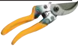
TIJERA PODA UNA MANO 144235 Mango de aluminio y recubierto en PVC, Ø máximo de corte 18 mm. 12'95
